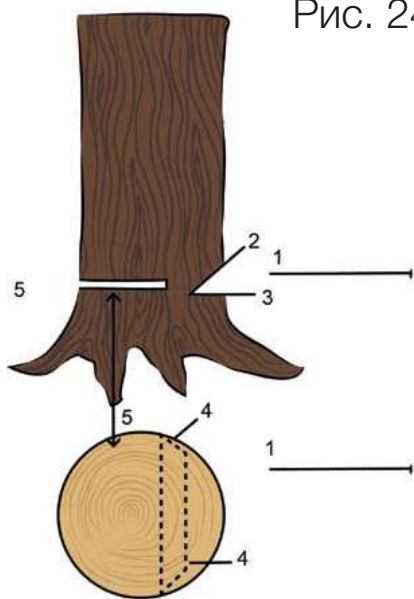
Рис. 24 Стандартный метод валки дерева (рис. 24)
